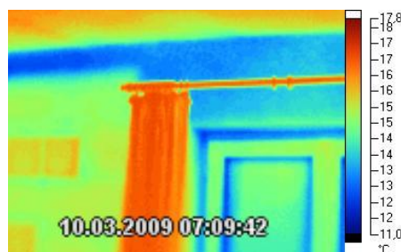
Wärmebrücke Betonsturz über Fenster
